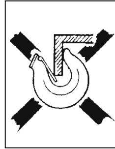
Fig 4 d Krokspetsen dessutom utsatt för böjpåkänning!
