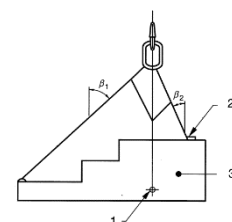
1 Tyngdpunkt 2 Hög påkänning i denna part 3 Last P
